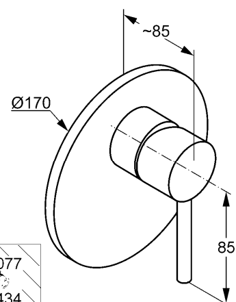
Размеры
